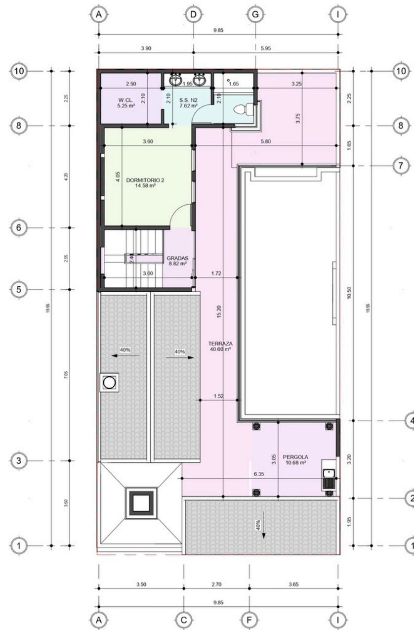
E9 SEGUNDO NIVEL - PLANTA DE AREAS ESC. 1 : 75
