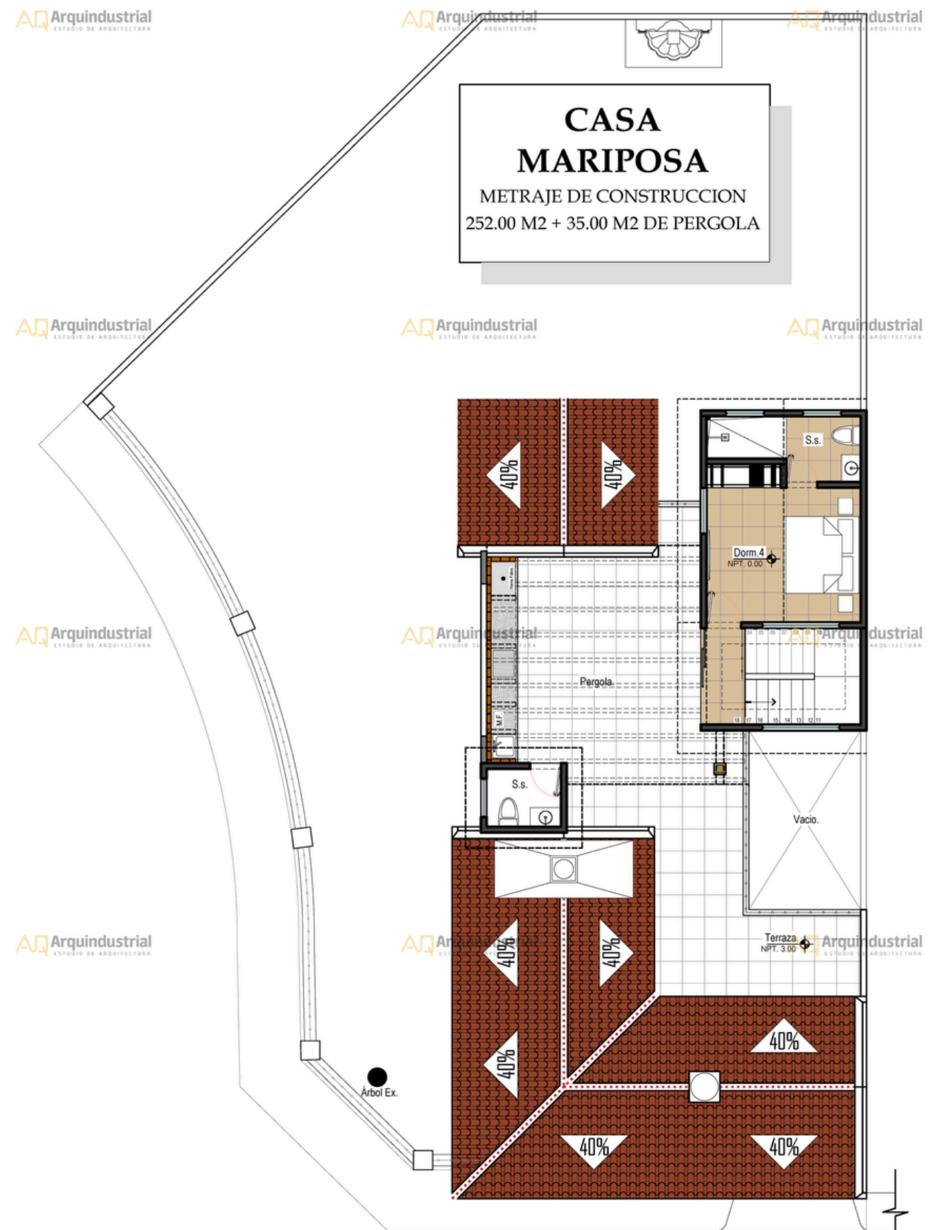
2 Planta de Techos Casa Mariposa - Sector G - Lote 11 ESCALA 1:100
