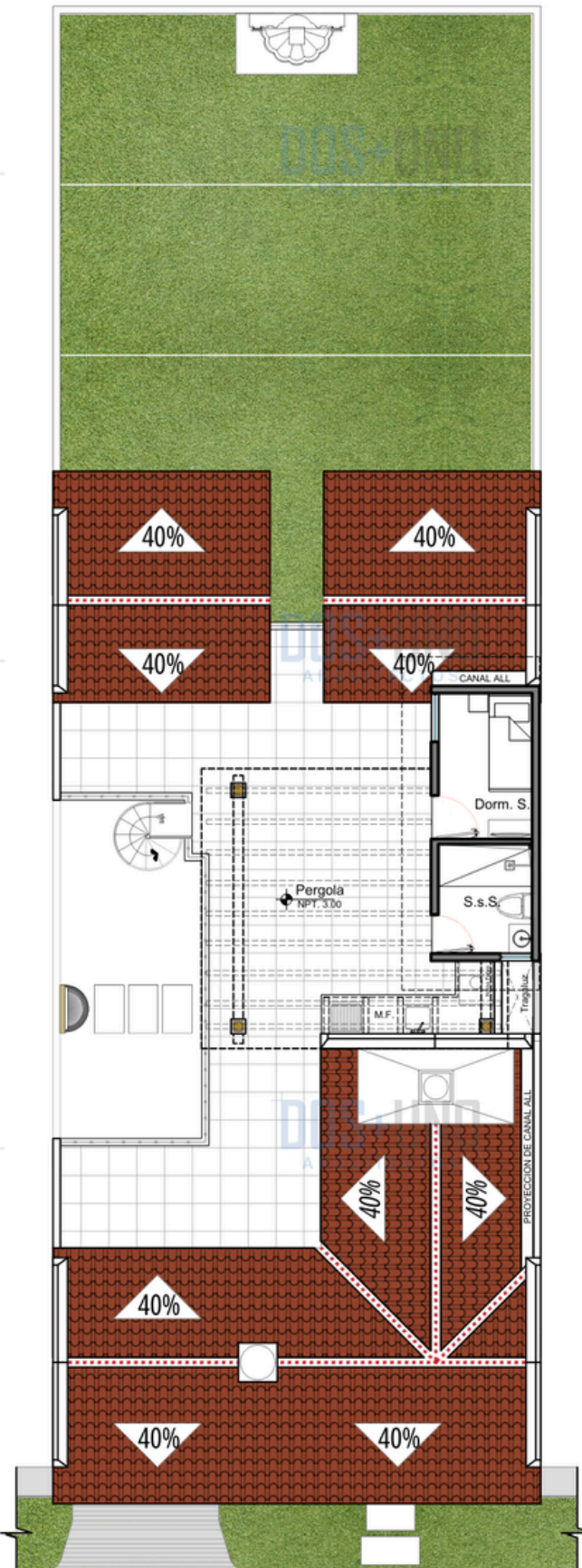
2 Planta de Techos Casa Mariposa - Sector K Lote 2 ESCALA 1:100
