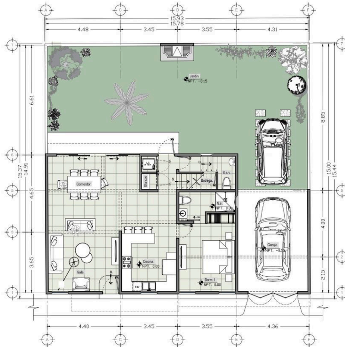
PLANTA DE ARQUITECTURA 1ER NIVEL ESC 1/100
