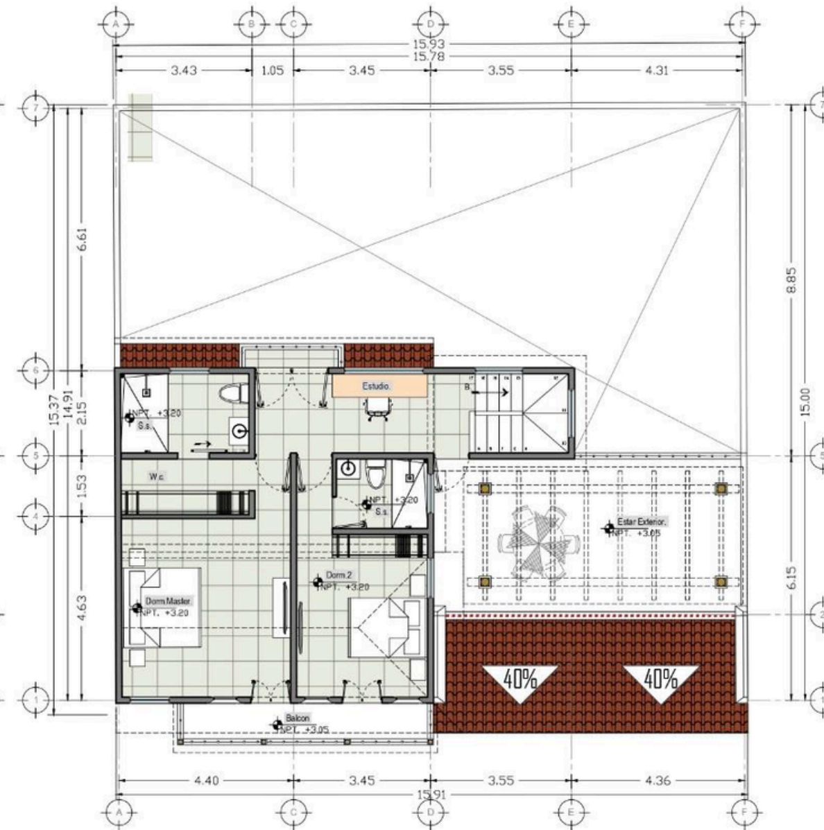
PLANTA DE ARQUITECTURA 2DO NIVEL ESC 1/100
