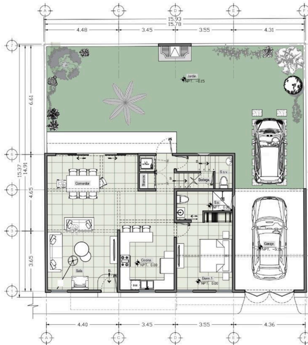
PLANTA DE ARQUITECTURA 1ER NIVEL ESC 1/100
