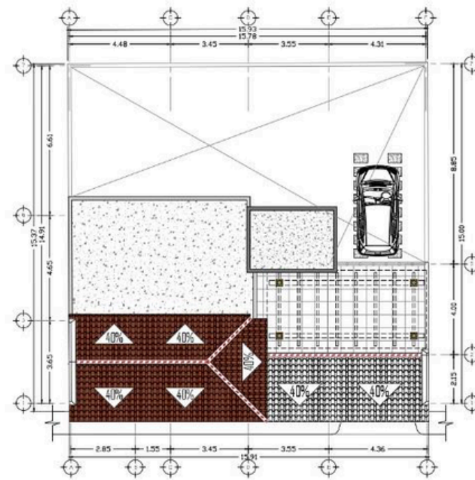
PLANTA DE CUBIERTAS ESC 1/125
