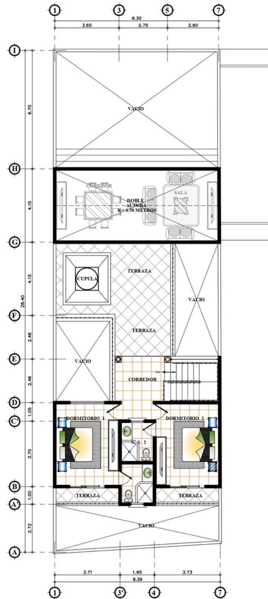
PLANTA ARQUITECTONICA.
