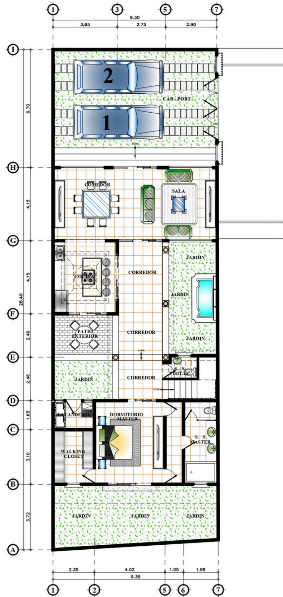
PLANTA ARQUITECTONICA.
