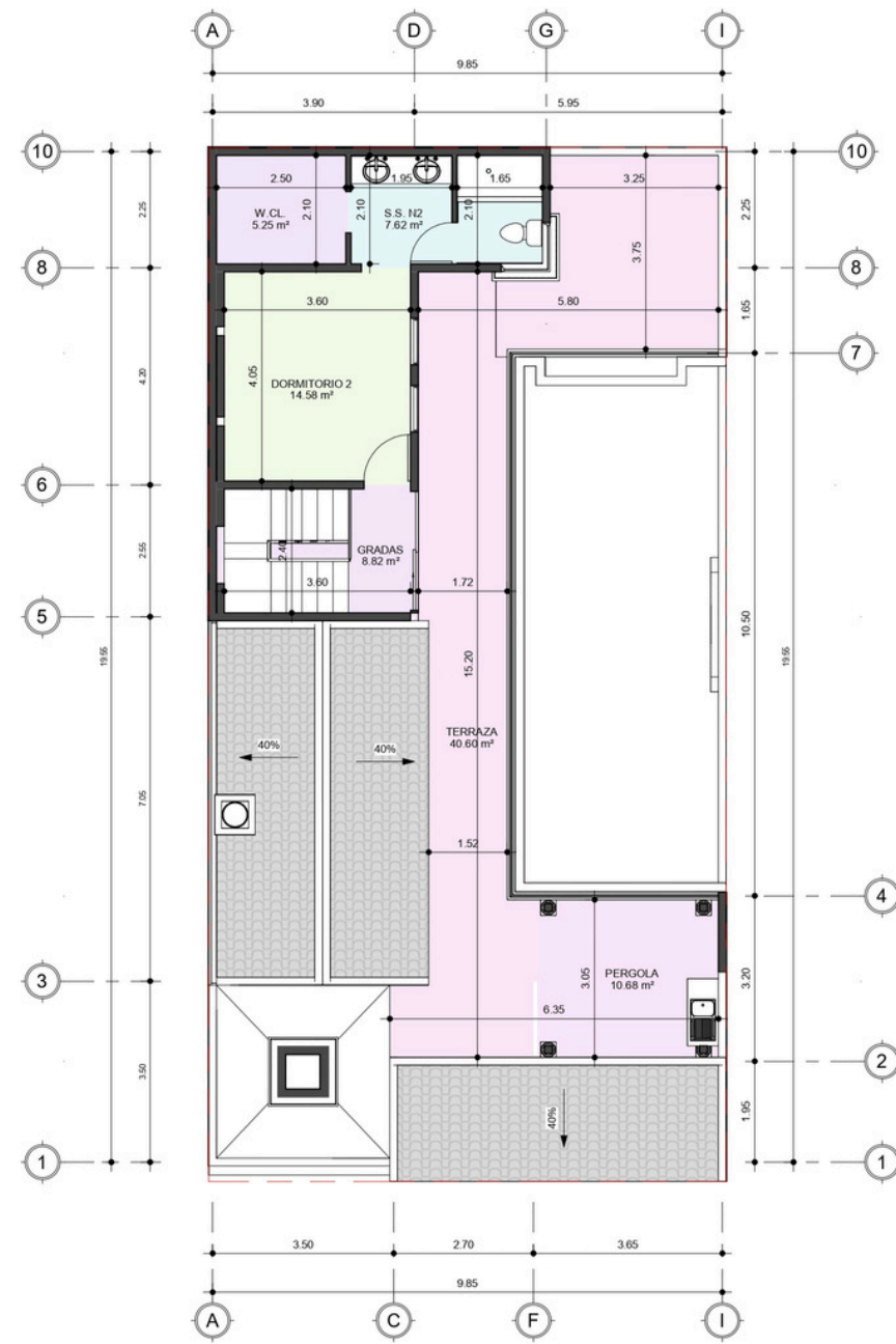
E9 SEGUNDO NIVEL - PLANTA DE AREAS ESC. 1 : 75
