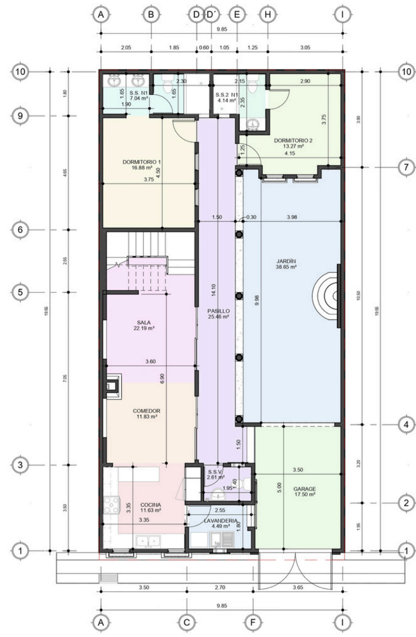
E1 PRIMER NIVEL - PLANTA DE AREAS ESC. 1 : 75
