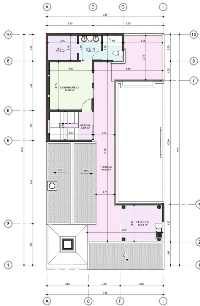
E9 SEGUNDO NIVEL - PLANTA DE AREAS ESC. 1:75
