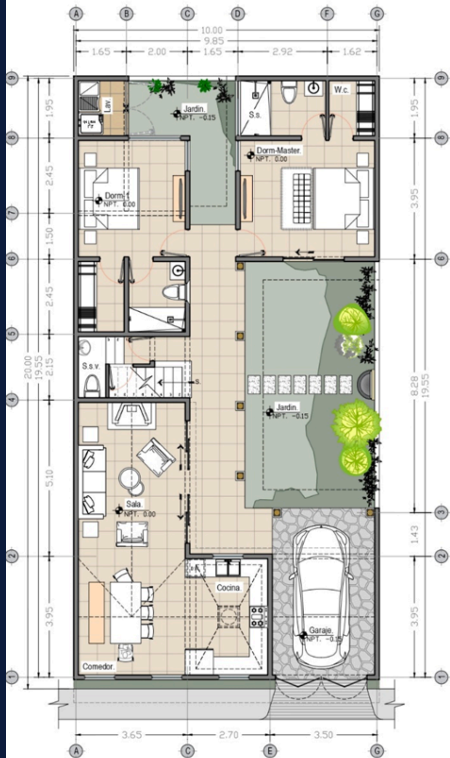
PLANTA DE ARQUITECTURA 1ER NIVEL ESC 1/100
