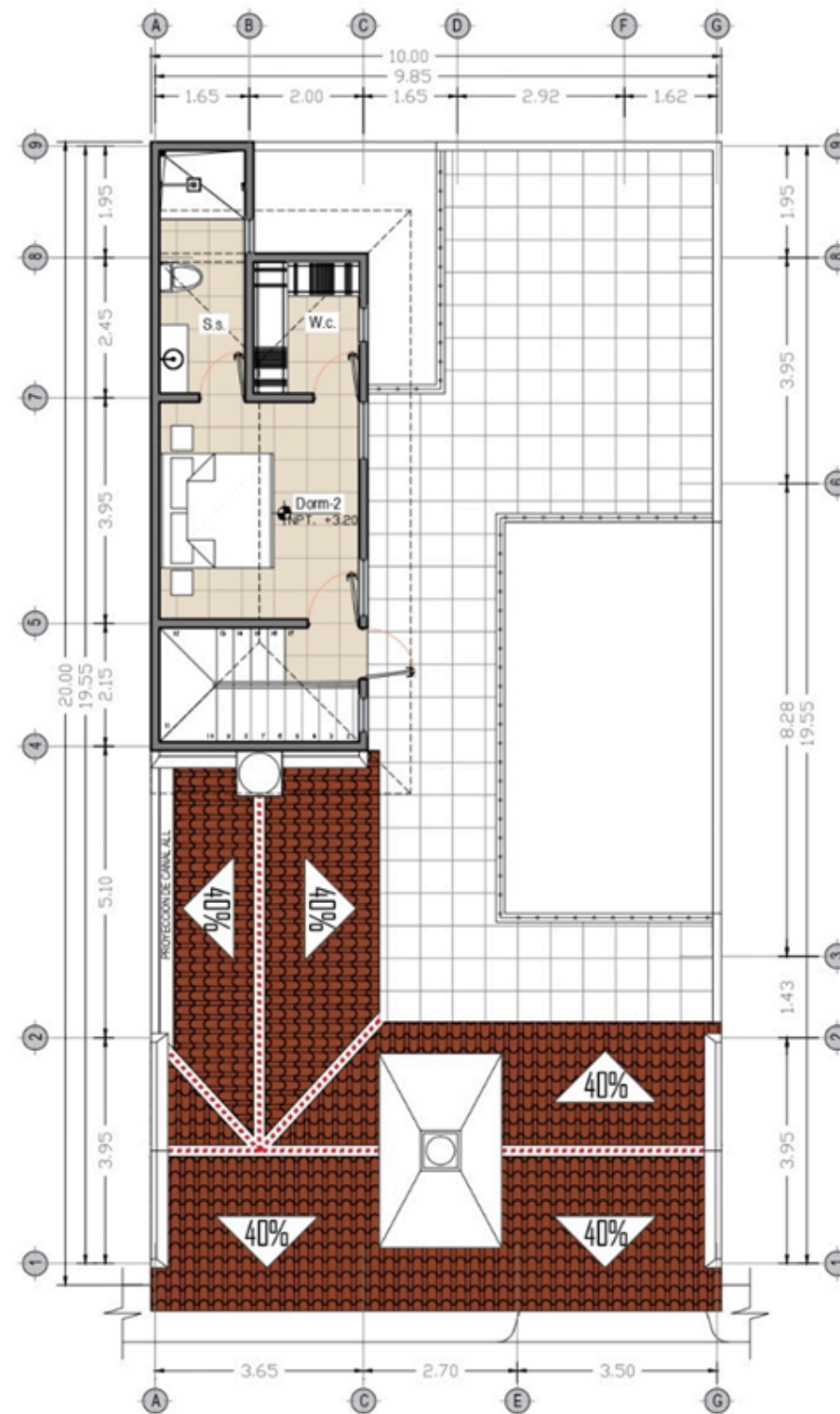
PLANTA DE CUBIERTAS ESC 1/100
