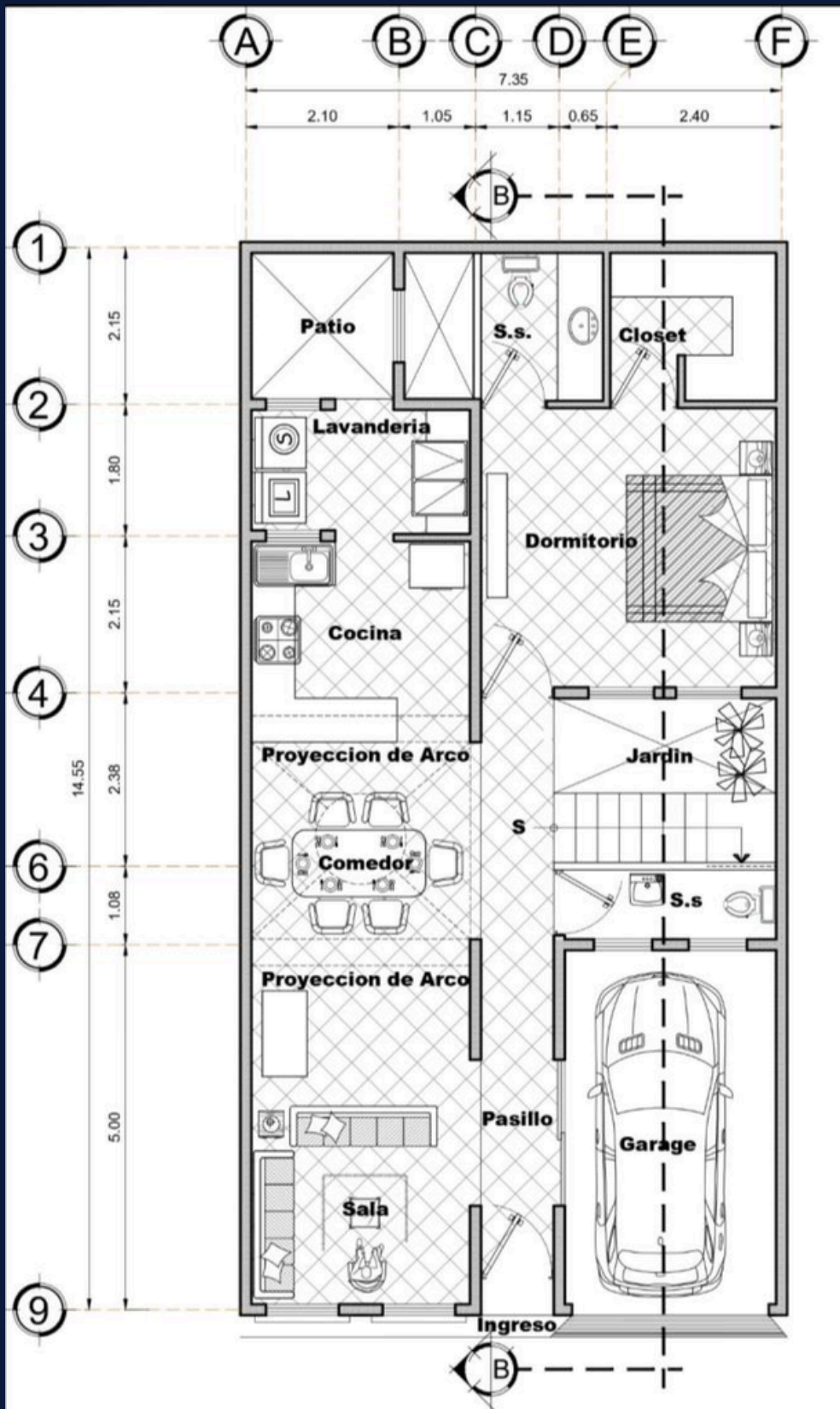
PLANTA BAJA AMUEBLADA Escala Grafica 1 M 2 M 3 M 4 M 5 M ESCALA 1/50
