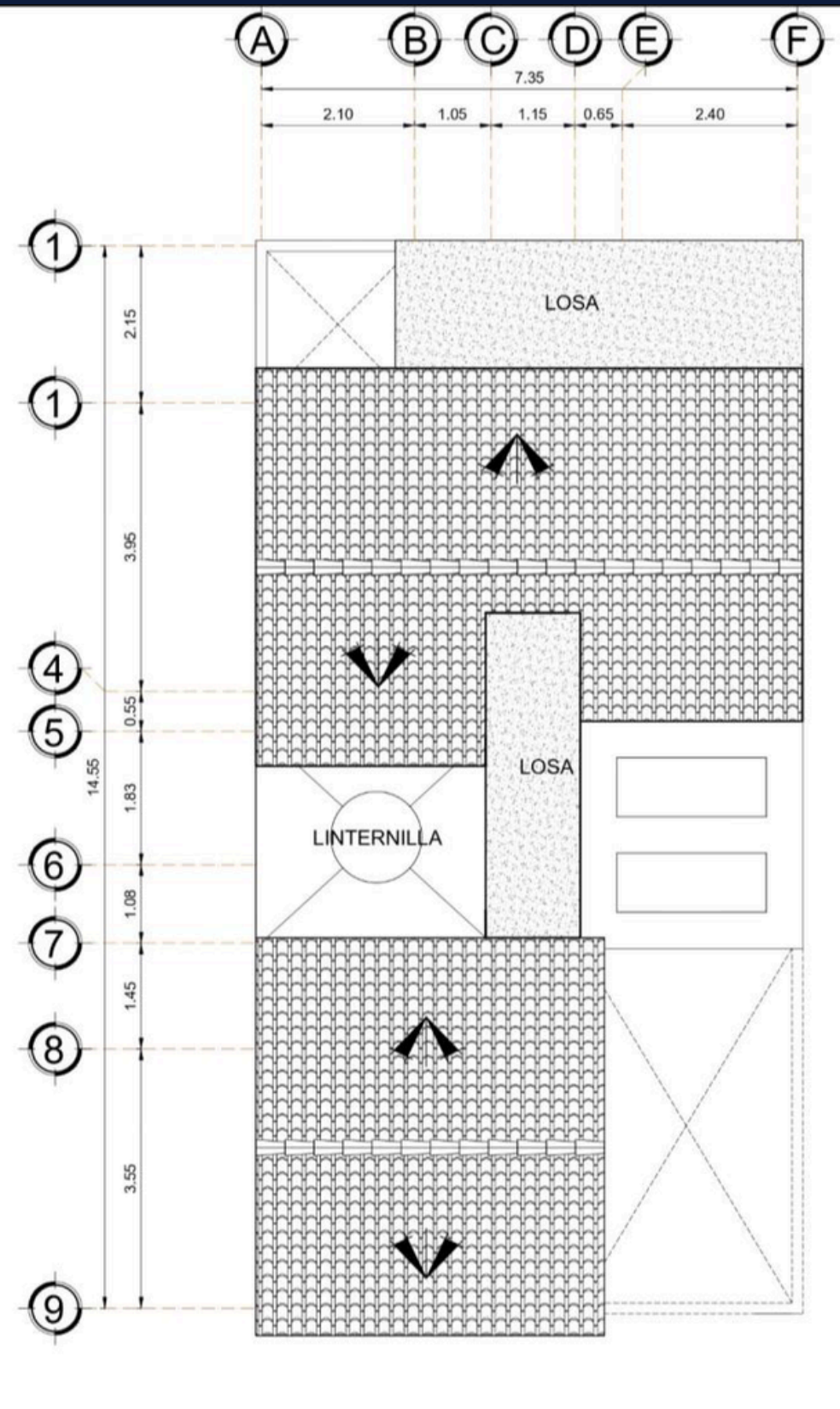
PLANTA DE TECHOS Escala Grafica 1 M 2 M 3 M 4 M 5 M ESCALA 1/50
