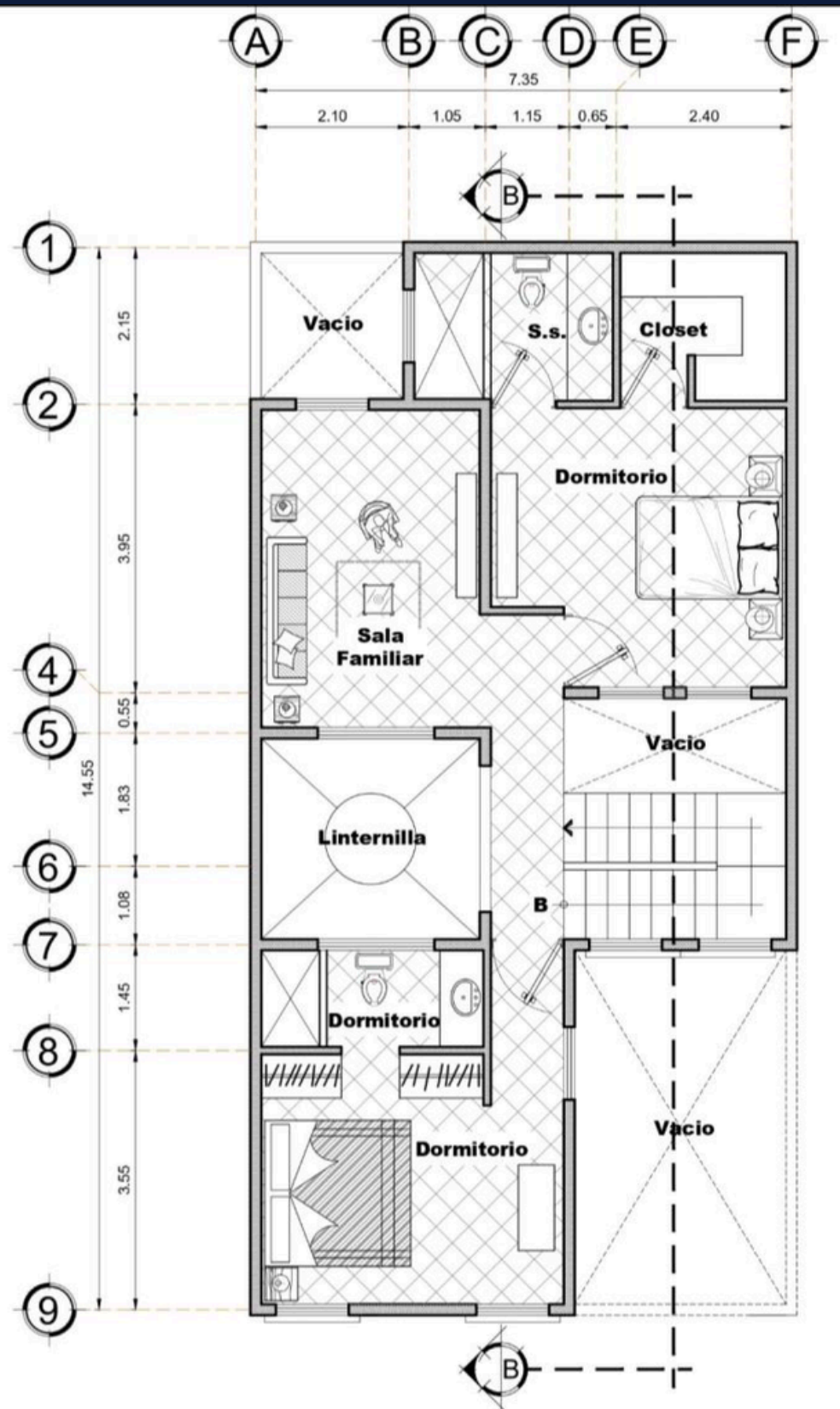
PLANTA ALTA AMUEBLADA Escala Grafica 1 M 2 M 3 M 4 M 5 M ESCALA 1/50
